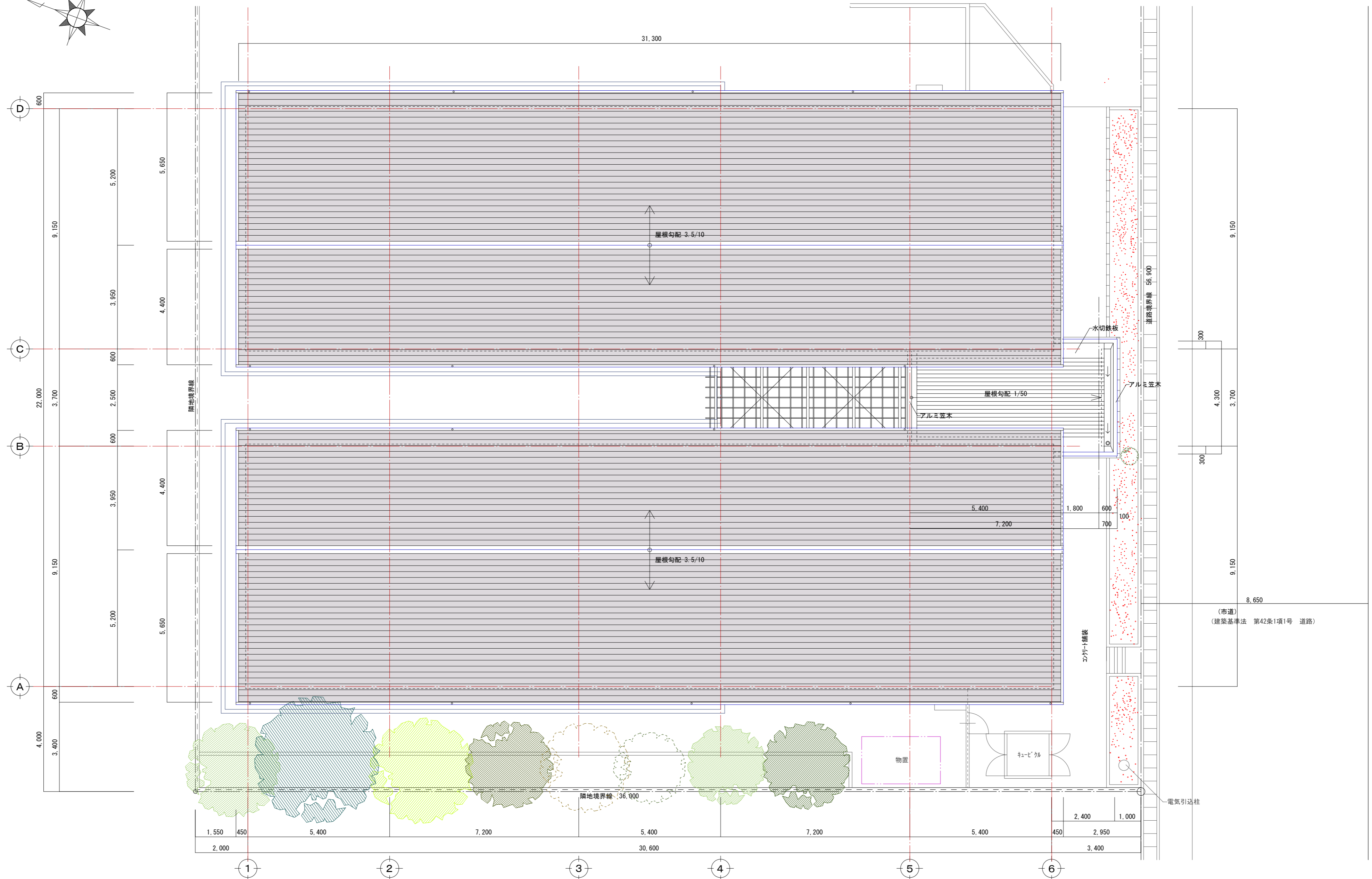
屋根伏図 S=1/100
